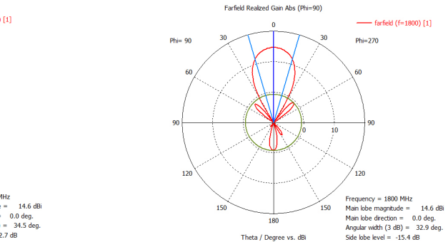
Диаграмма направленности Е-плоскость
