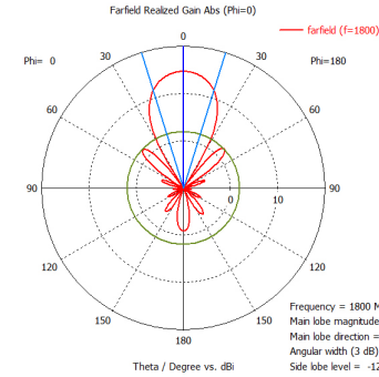
Диаграмма направленности Н-плоскость
