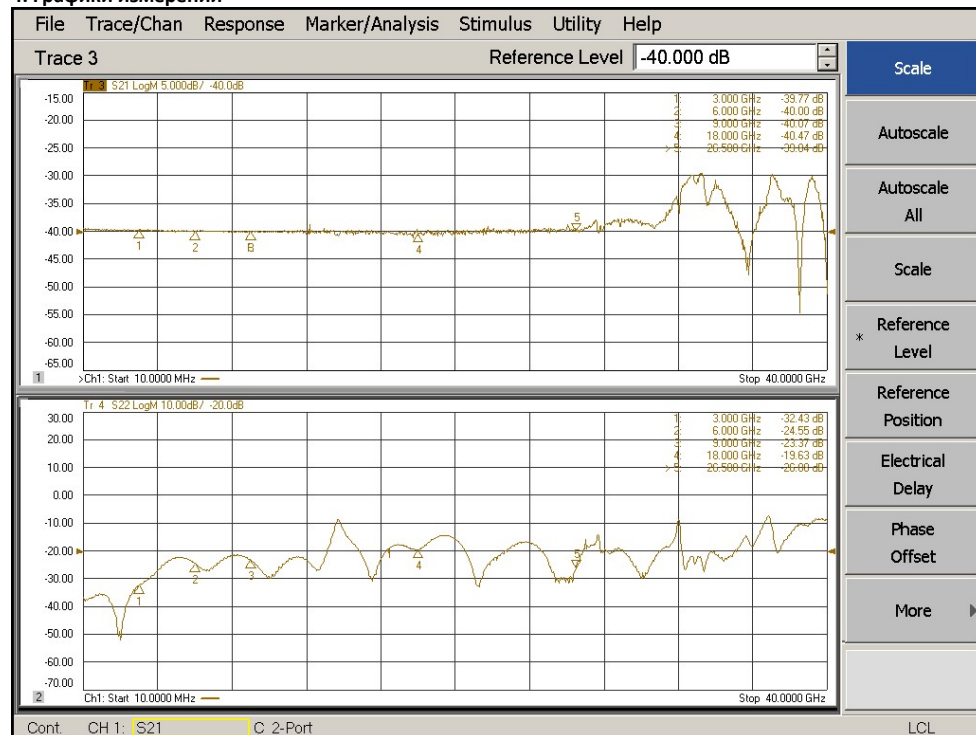
Графики для АЧХ при отсчётом уровне равном -40 дБ и -20 дБ
