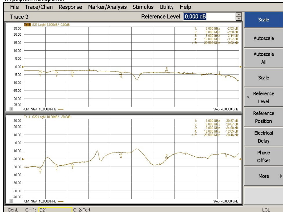
Графики для АЧХ при отсчётном уровне равном 0 дБ и -20 дБ
