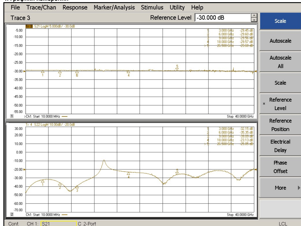
Графики для АЧХ при отсчётном уровне равном -30 дБ и -20 дБ
